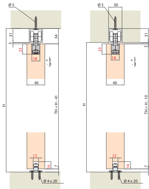
Montage aufgesetzt
