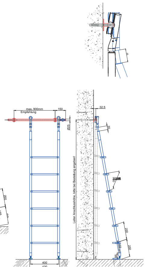
Beispiel Modell SL 6085 mit Edelstahlstufen
