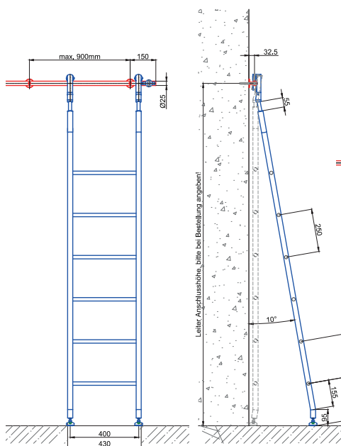
Beispiel Modell SL 6085 mit Edelstahlsprossen
