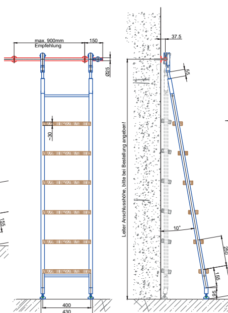
Beispiel Modell SL 6085 mit Holzstufen
