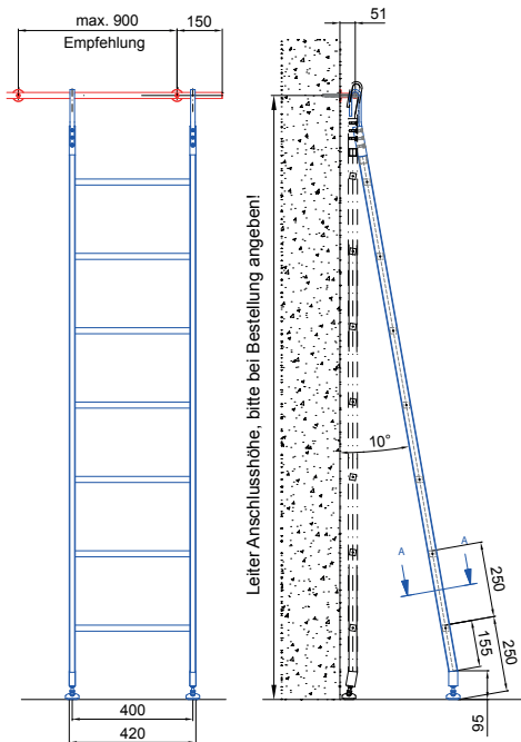
Beispiel Modell SL 6005 AK mit Edelstahlspinnen
