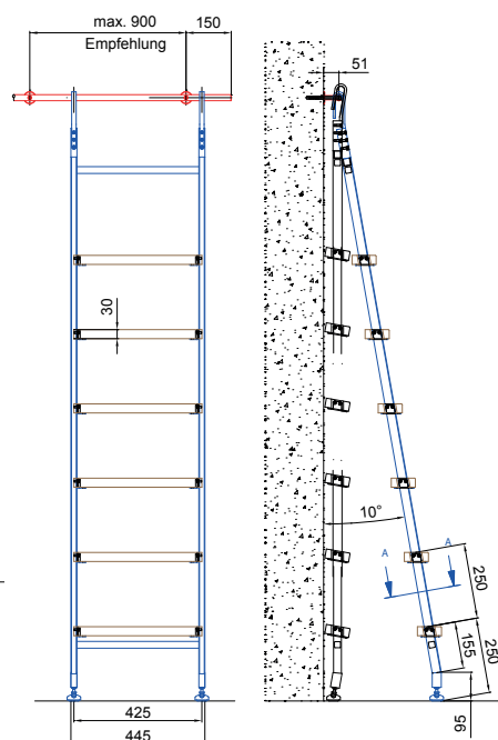
Beispiel Modell SL 6005 AK mit Holzstufen
