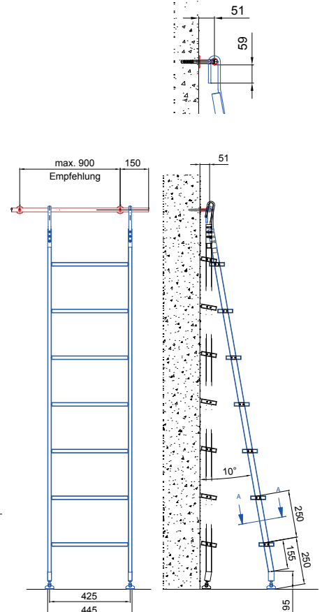
Beispiel Modell SL 6005 AK mit Edelstahlstufen
