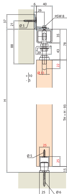
Wandmontage mit Laufschiene Stahl, U-Führungsschiene und Bodenführung mit Rolle.
