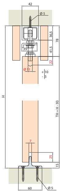
Deckenmontage mit Laufschiene Alu
