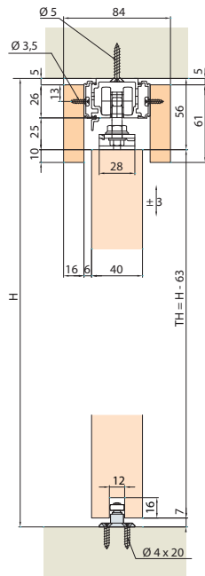
Deckenmontage mit Combi-Laufschiene, Clip-Teil / Holzblende.
