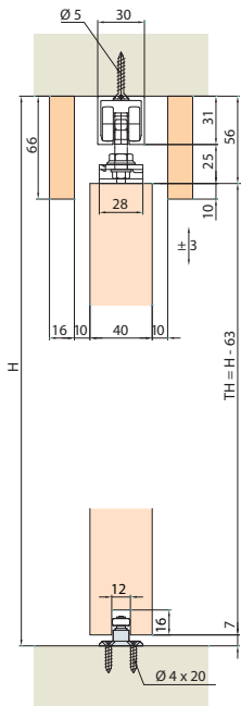
Deckenmontage mit Einfachlaufschiene.
