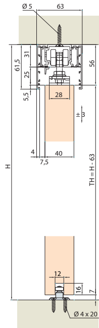
Deckenmontage mit Combi-Laufschiene, Clip-Teil / Clip-Blende Alu.
